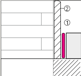
Installazione su massetto Shower tray installation on screed
