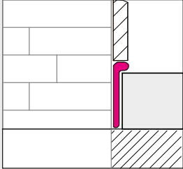
Installazione sotto piastrella Shower tray installation under tiles
