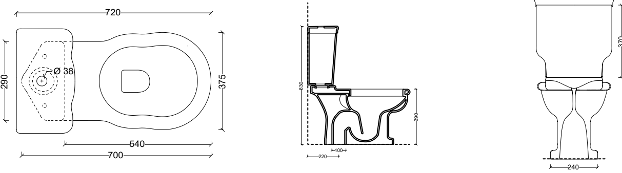
28290101 Vaso Monoblocco BOHEME scarico a parete
