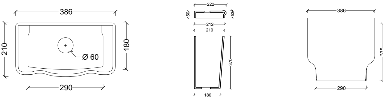
28300101 cassetta monoblocco BOHEME
