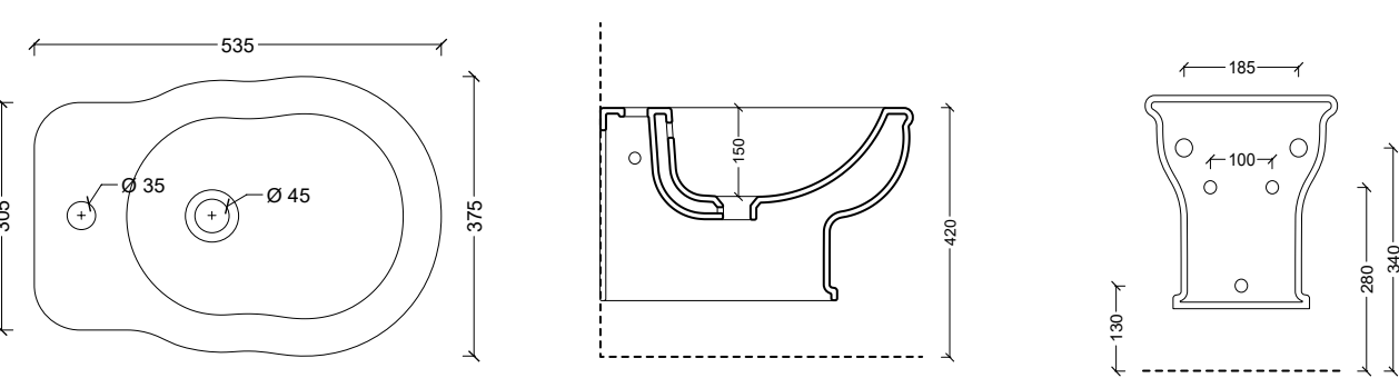
28280101 Vaso Monoblocco BOHEME scarico a terra
