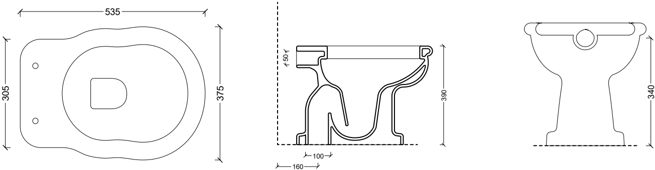
28210101 Vaso a terra BOHEME scarico a parete
