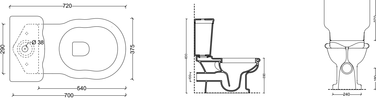
28300101 cassetta monoblocco BOHEME
