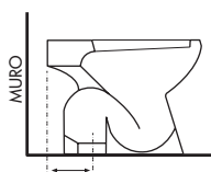
VANTALW Vaso monoblocco a terra VAMPALW Vaso monoblocco s/parete CSMZALW Cassetta monoblocco
